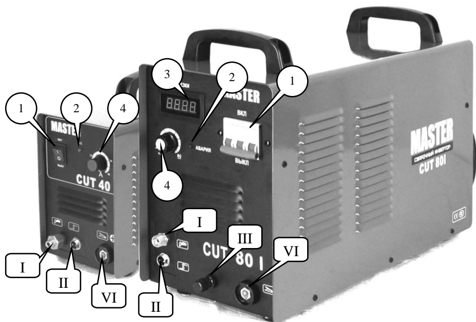
Рис.1. Органы управления и индикации аппаратов.
